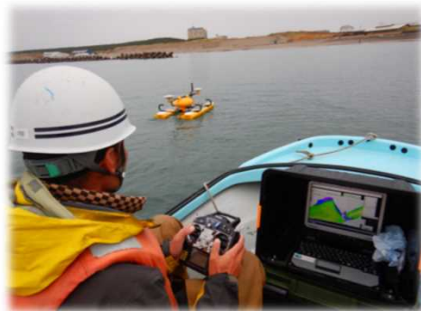
NMB（ナローマルチビーム）測量
